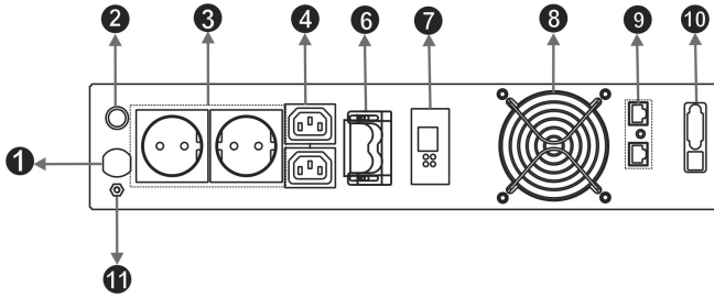
شکل ۱۸: نمای پشت یوپی‌اس‌های سری DSS3000X-RT-48V و DSS2000X, DSS1500X
