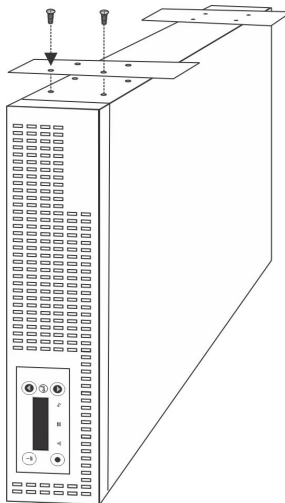
شکل ۱۵: بستن پلایت‌های فلزی به DSS1500B-RT
