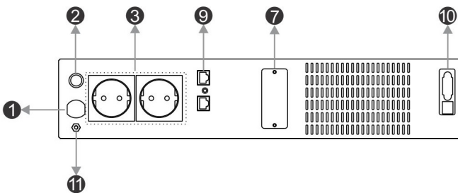
شکل ۲۰: نمای پشت یوپی‌اس‌های سری DSS1500B
