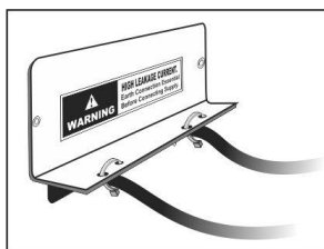
شکل ۲۰: نحوه‌ی محکم کردن کابل‌ها به درپوش L شکل ترمینال ورودی-خروجی
