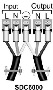
شکل ۱۹: اتصال کابل‌های ورودی و خروجی
