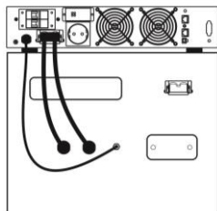
شکل ۸: SDC1500-RT
