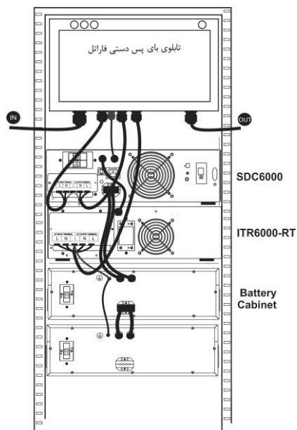
شکل ۱۴-د: یوپی اس SDC6000، ترانسفورمر ایزوله و کابینت باتری و تابلوی بای پس
